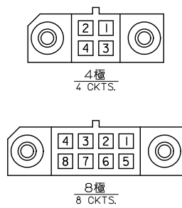
回路レイアウト図
