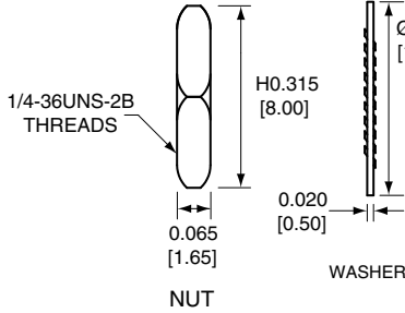
NUT
