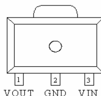
SOT-89-3LB
