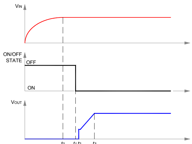
Fig. G: Startup scenario #2.
