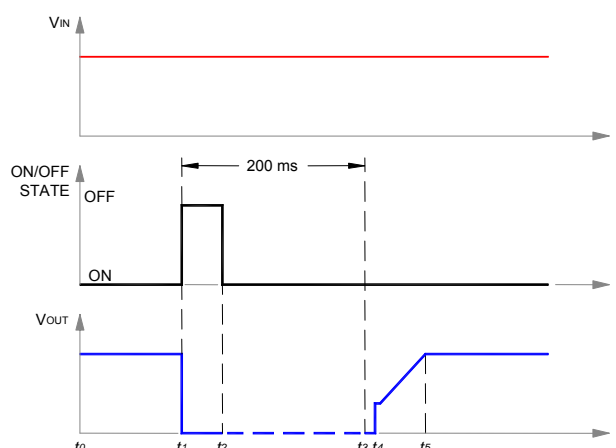
Fig. H: Startup scenario #3.
