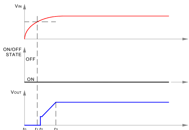
Fig. F: Startup scenario #1.
