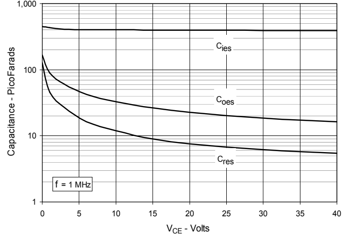
Fig. 10. Capacitance
