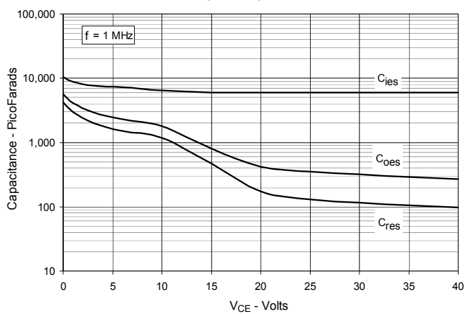
Fig. 9. Capacitance
