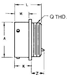
Solder KPT01/MS3111
