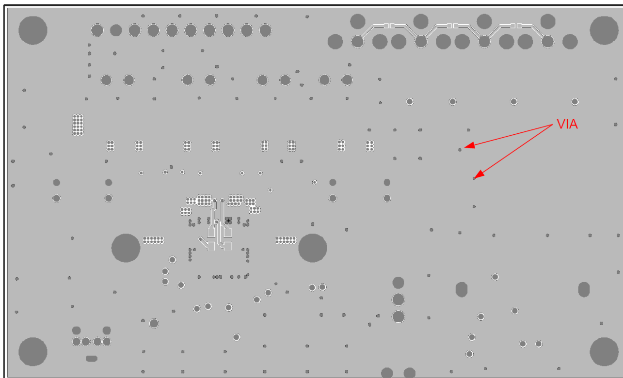
Figure 26. Bottom Layer
