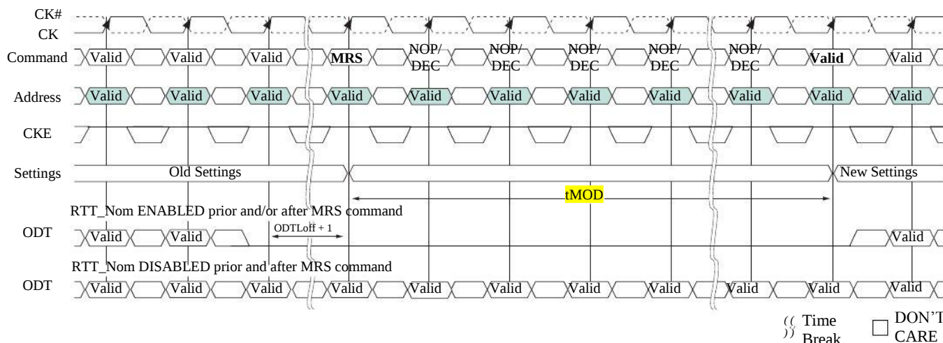
Figure 2.3.1b tMOD Timing
