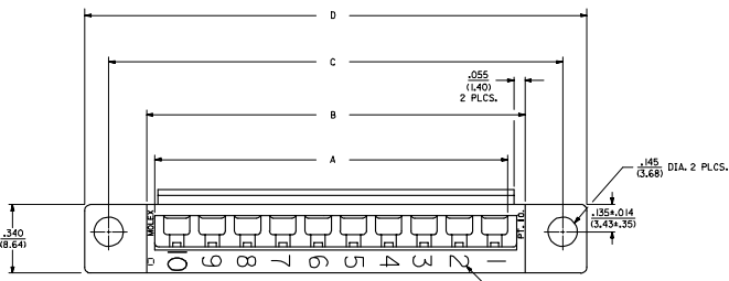
VIEW A-A
