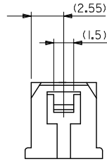
2極の場合 IN CASE OF 2 CIRCUIT HSG.
