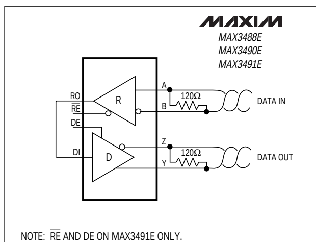
Figure 21. Line Repeater for MAX3488E/MAX3490E/MAX3491E
