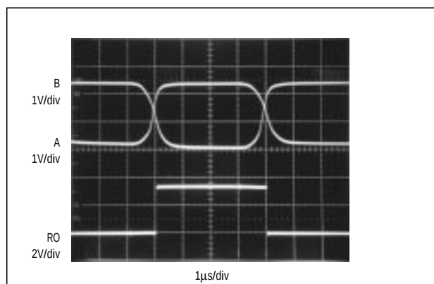
Figure 18. MAX3483E/MAX3488E Receiver Propagation Delay
