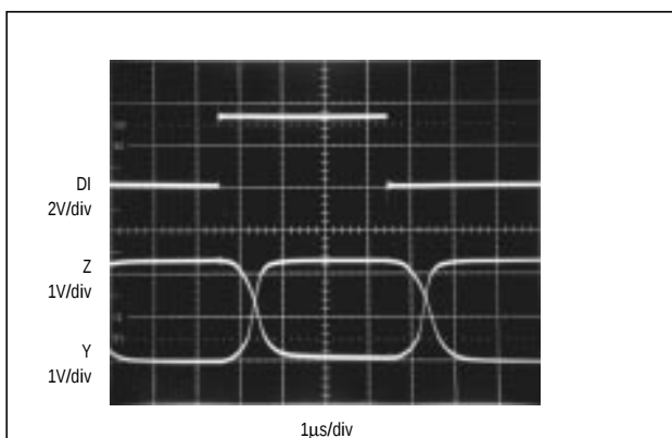
Figure 17. MAX3483E/MAX3488E Driver Propagation Delay
