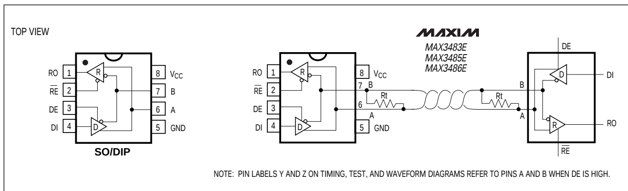
Figure 1. MAX3483E/MAX3485E/MAX3486E Pin Configuration and Typical Operating Circuit
