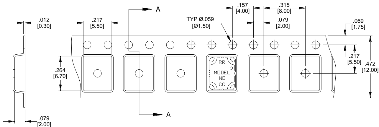
SECTION A-A
