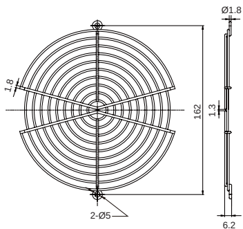
FG-17B For 172mm Fan
