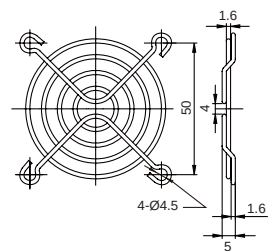
FG-06 For 60mm Fan
