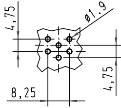
Lochbild / pinhole pattern
