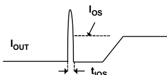
Figure 27. Output Short-Circuit Parameters
