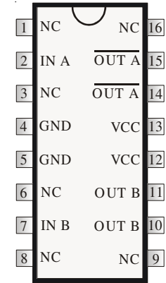
16 Pin SOIC IXDF404SI-16
