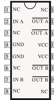
16 Pin SOIC IXDI404SI-16
