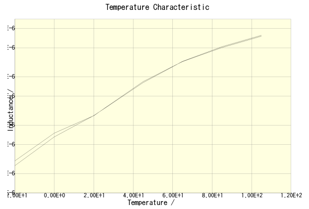
CLF10040T-1R5N-CA(DC = 0A)
