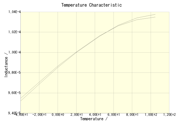
CLF12555T-101M-CA(DC = 0A)
