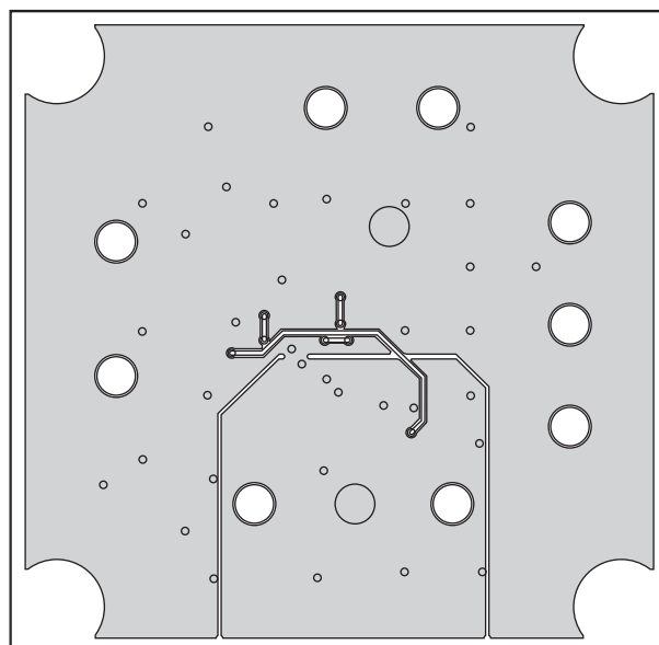
Bottom Side(Layer 4)
