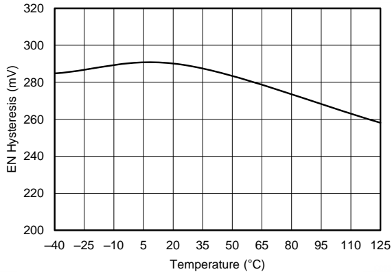
Figure 21. EN Hysteresis
