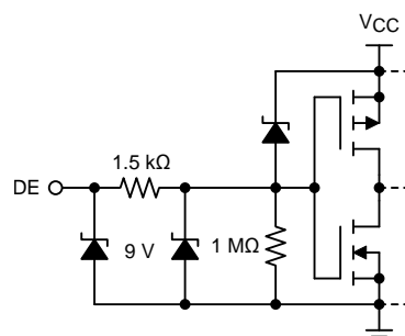
Figure 26. DE Input
