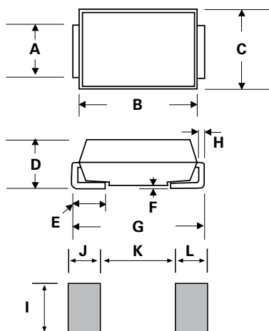
DO-214AC (SMA)
