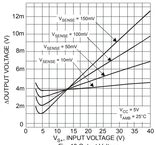
Fig. 10 Output Voltage
