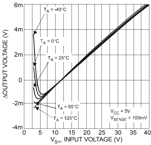
Fig. 11 Output Voltage
