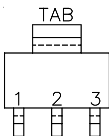
SOT-223
