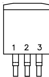
TO-263-3
