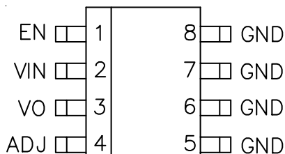
SO-8
