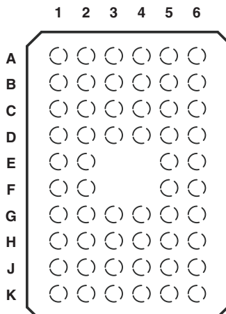
GQL/ZQL PACKAGE (TOP VIEW)
