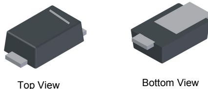
POWERDI323
