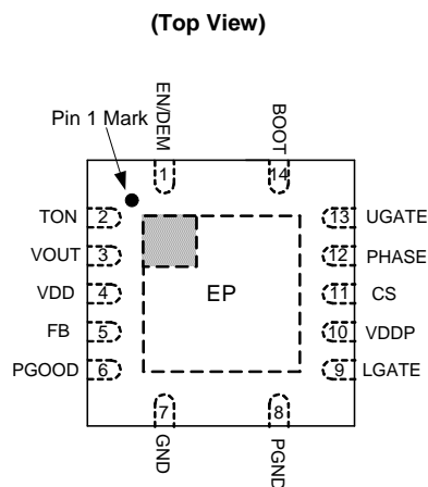
U-QFN3535-14
