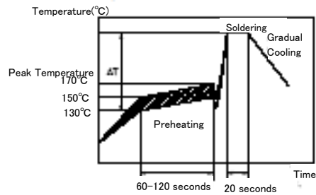
Vapor Reflow
