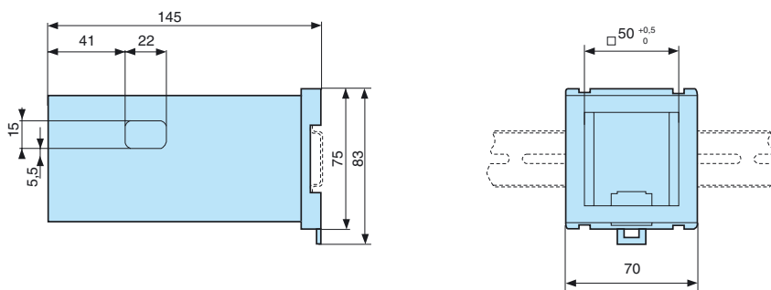
26546841 - DIN rail adaptor
