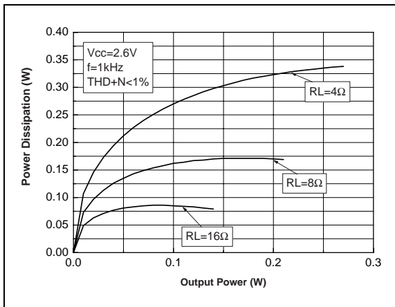
Fig. 19 : Power Dissipation vs Pout
