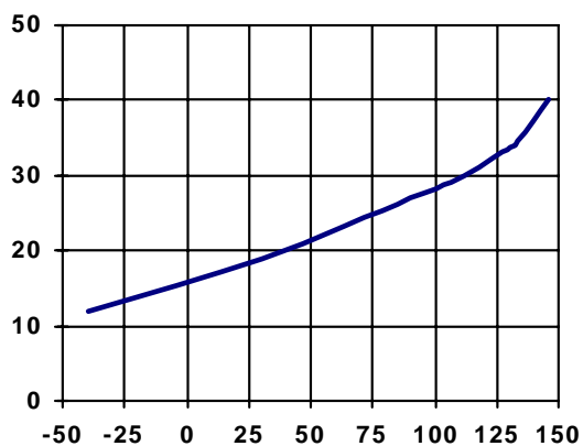
Figure 7 - Iccoff (µA) vs Tj (°C)
