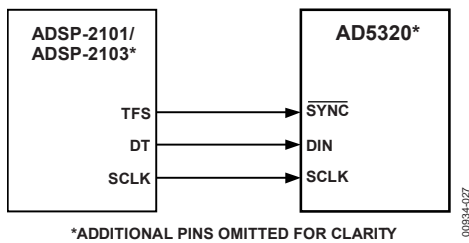
Figure 28. AD5320 to ADSP-2101/ADSP-2103 Interface
