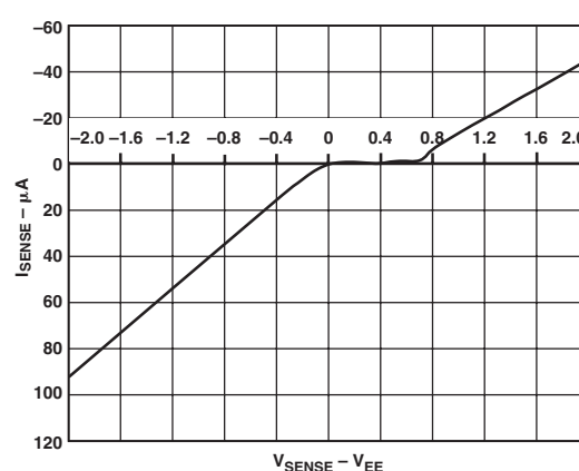
TPC 18. I_{SENSE} vs. (V_{SENSE} - V_{EE})
