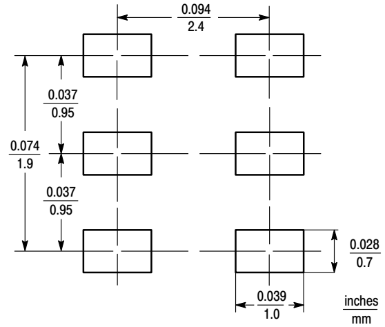
SOT23-6
