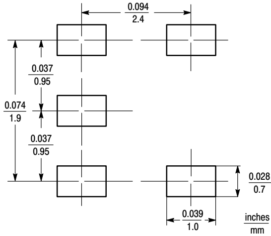
SOT23-5
