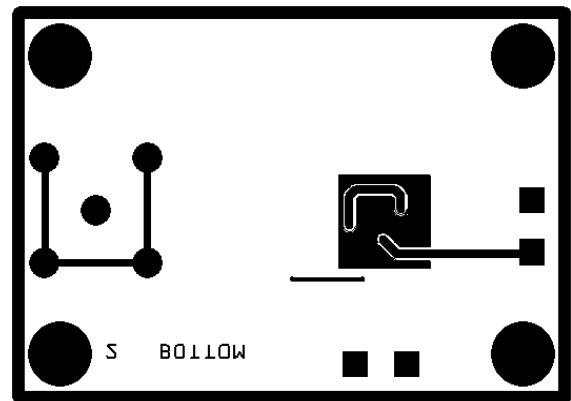
Bottom Layer
