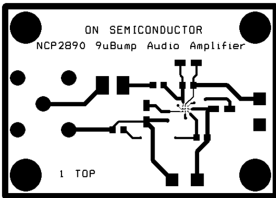
Top Layer
