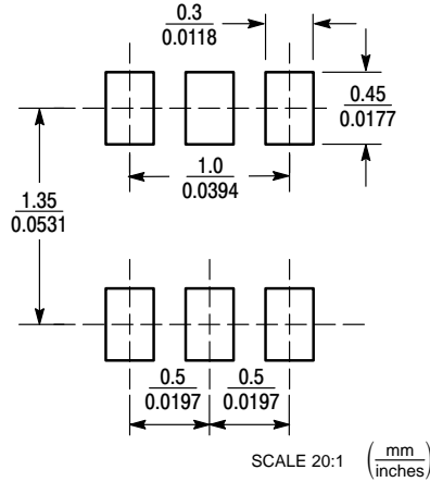
SOT-563
