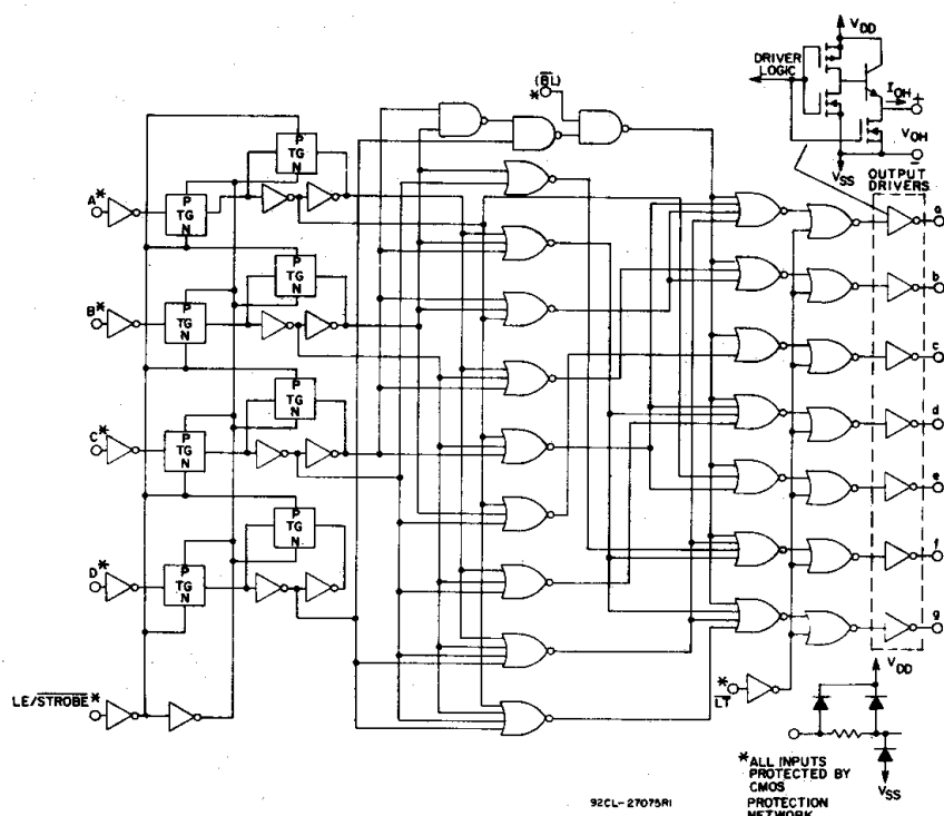
Fig. 8 - Logic diagram.
