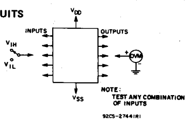
Fig. 10 - Input voltage.
