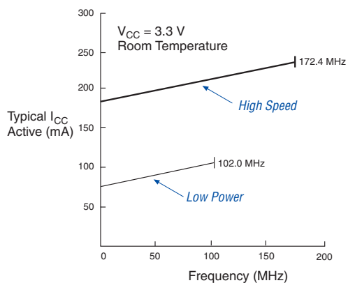
EPM3256A
