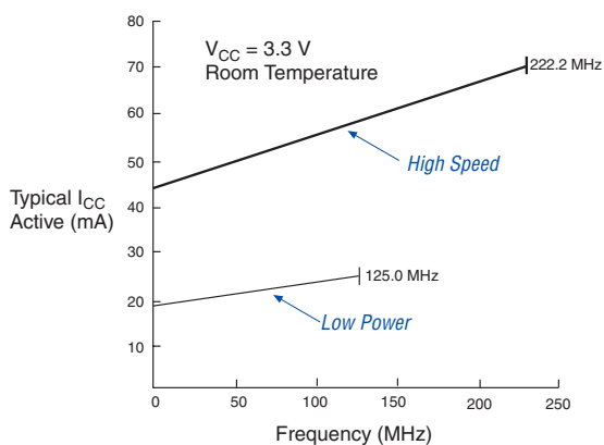
EPM3064A
