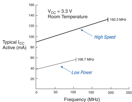
EPM3128A
