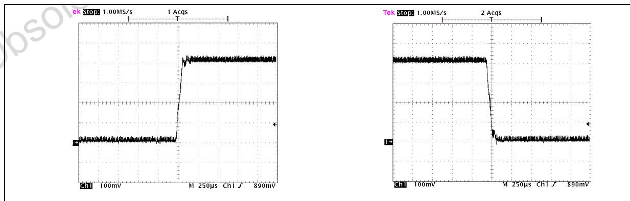
Figure 27. Dynamic VID Response
