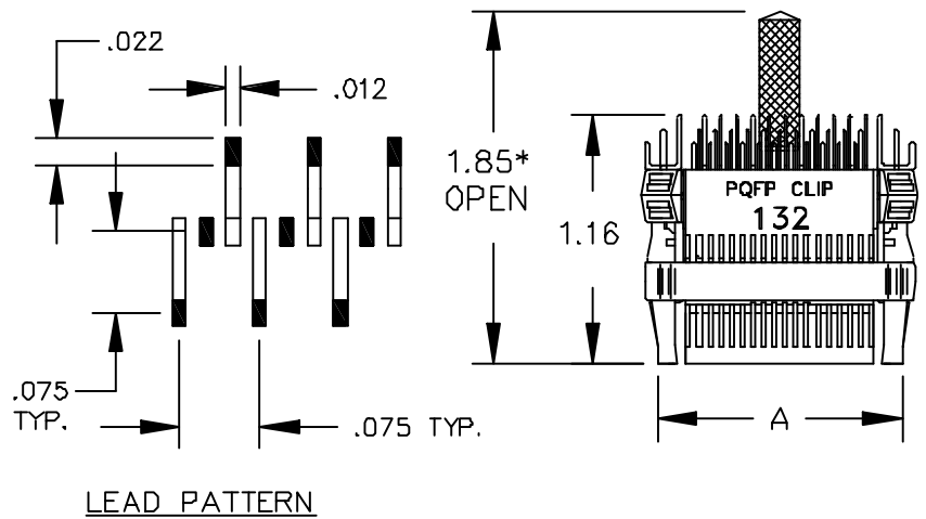
132 PIN JEDEC CHIP
