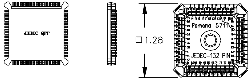
132 PIN JEDEC CHIP
