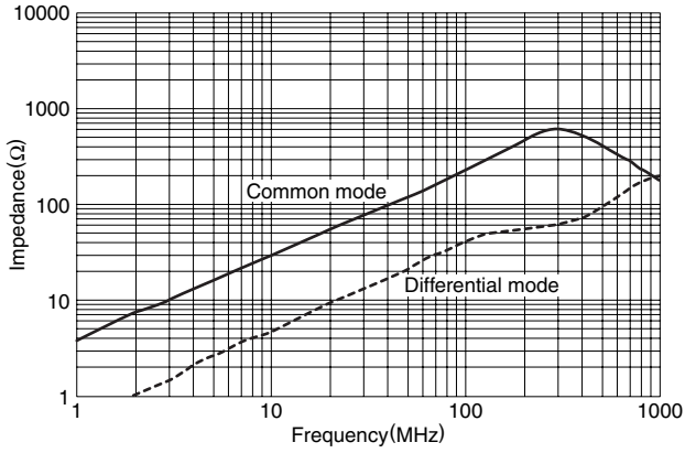
ACM4520-231-2P
