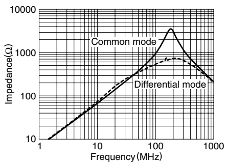
ACM1513-551-2PL-TLHF
