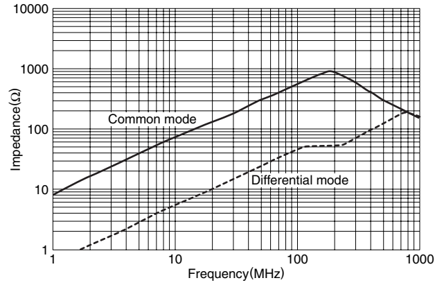
ACM4520-421-2P
