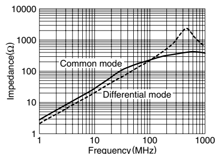
ACM1211-701-2PL-TL01
