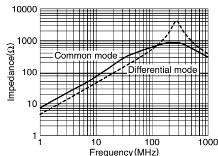
ACM1513-551-2PL-TLHF
