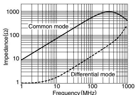
ACM3225-601-2P
