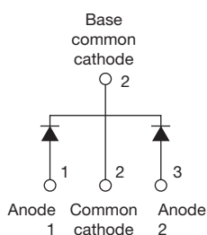
VS-MURB1020CTPbF
