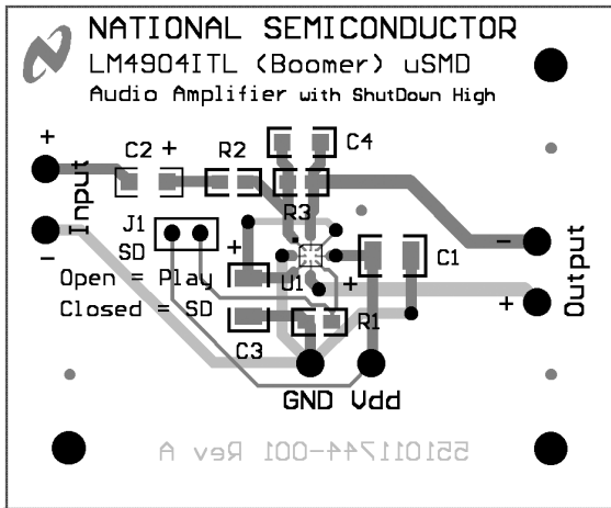
Top Layer
