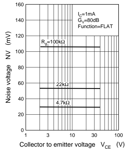
NV - V_{CE}
