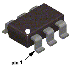
SuperSOT™-6
