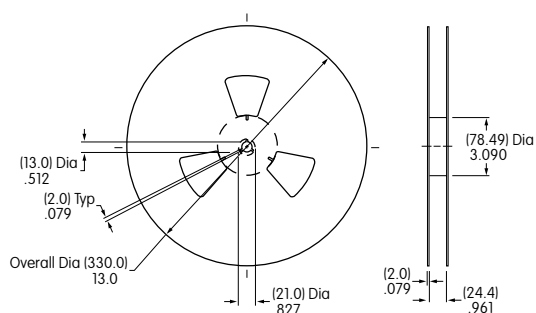
Reel Dimensions
