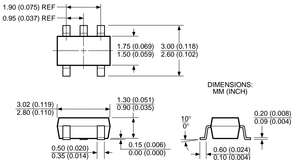
SOT-23-5 (M5)
