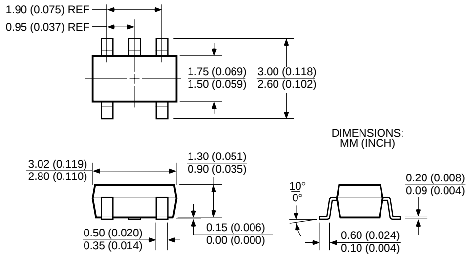
SOT-23-5 (M)
