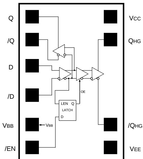
SY10/100EL16VDXC DIE
